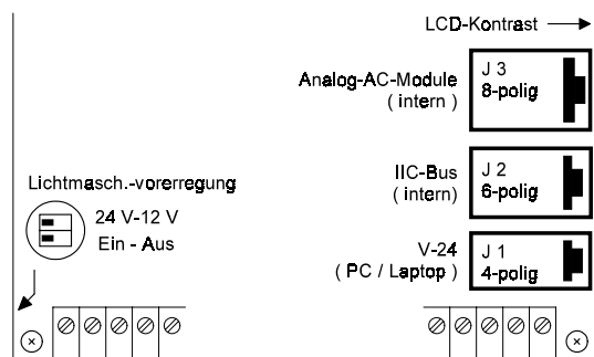
Abb.8: Kodierung Lichtmaschinen-vorerregung, Schnittstellen
